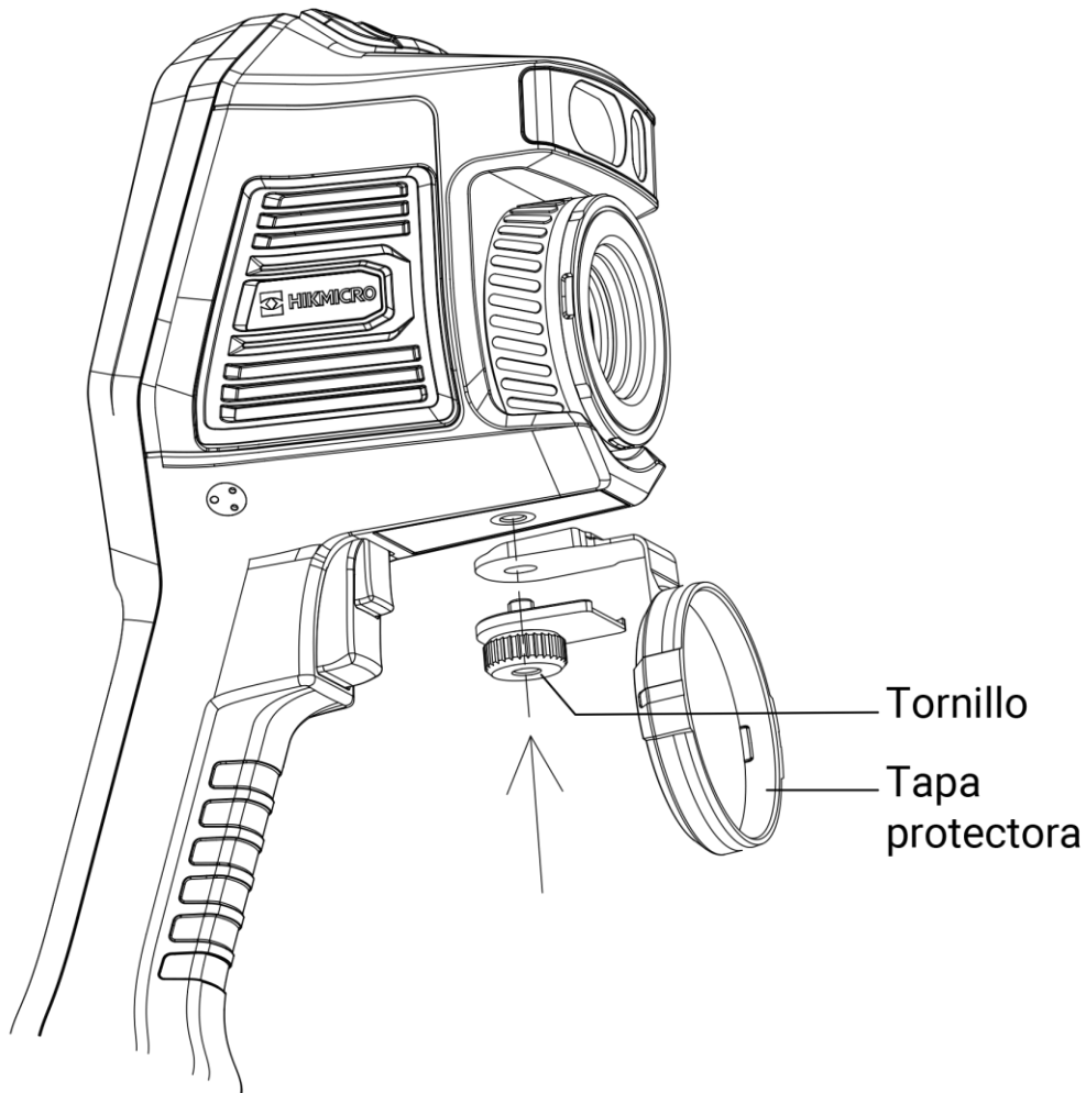
Figura 2-5 Fijar la cubierta protectora
