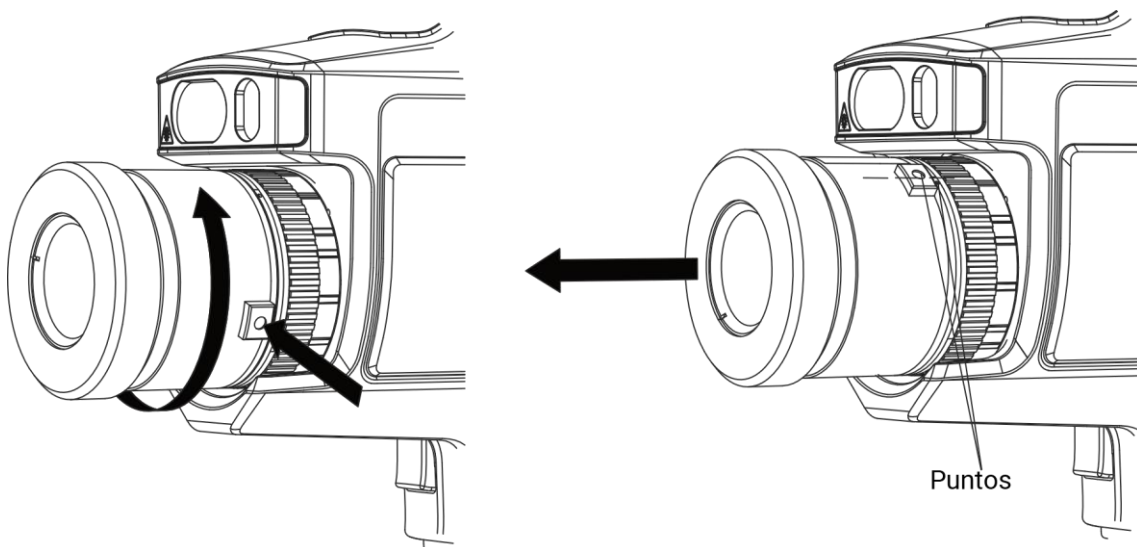
Figura 2-9 Desmontaje de la lente
