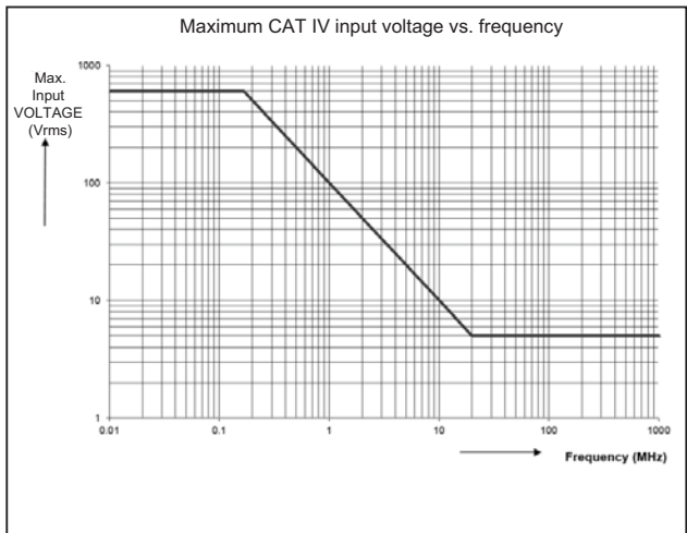
Figura 16. Manipulación segura: Tensión máx. entre la referencia del Instrumento de comprobación y la puesta a tierra
