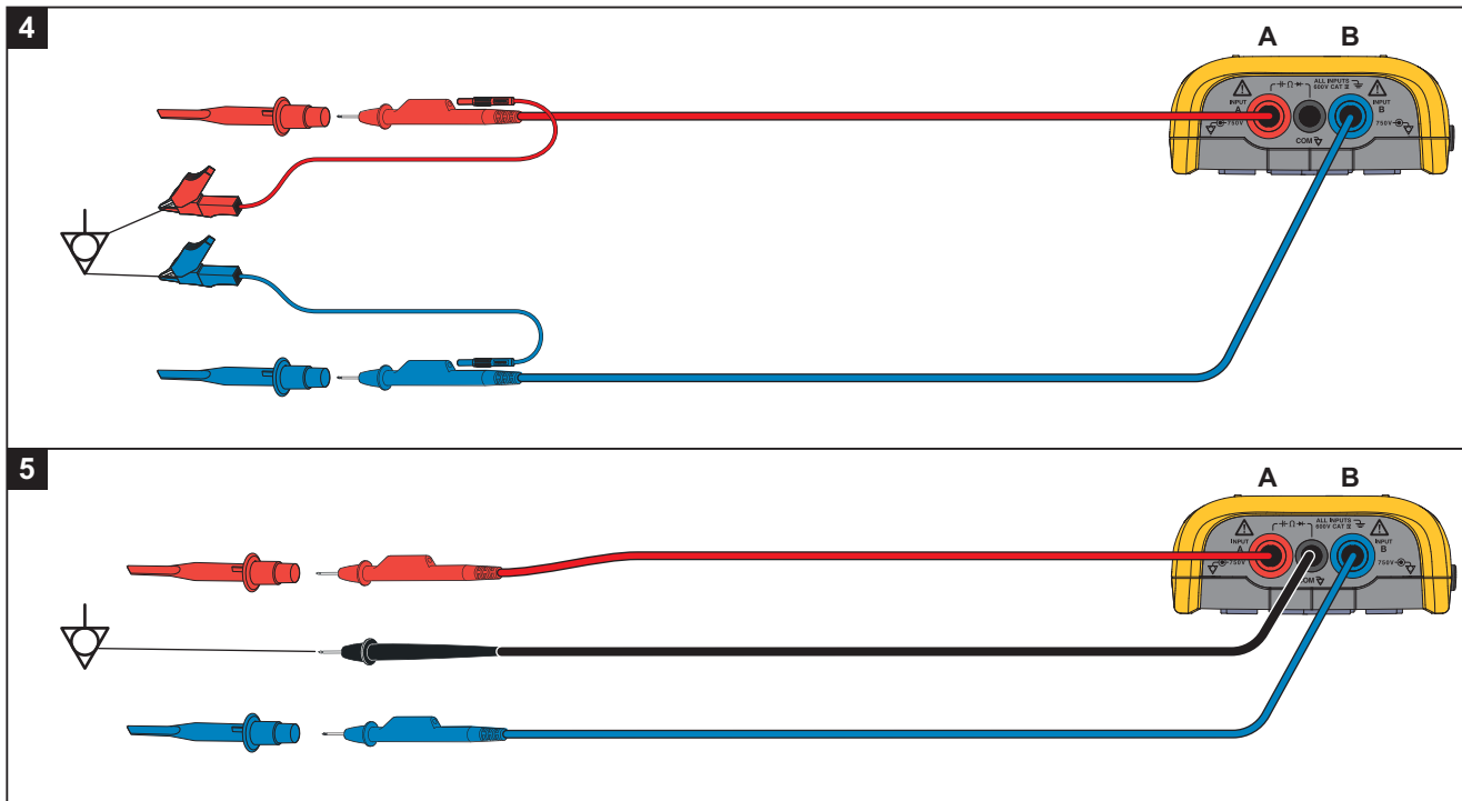
Figura 8. Configuración de conexión a masa correcta
