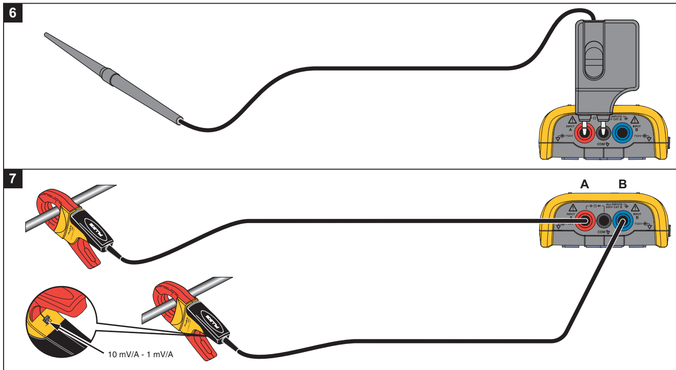
Figura 9. Configuración de medición de temperatura y corriente
