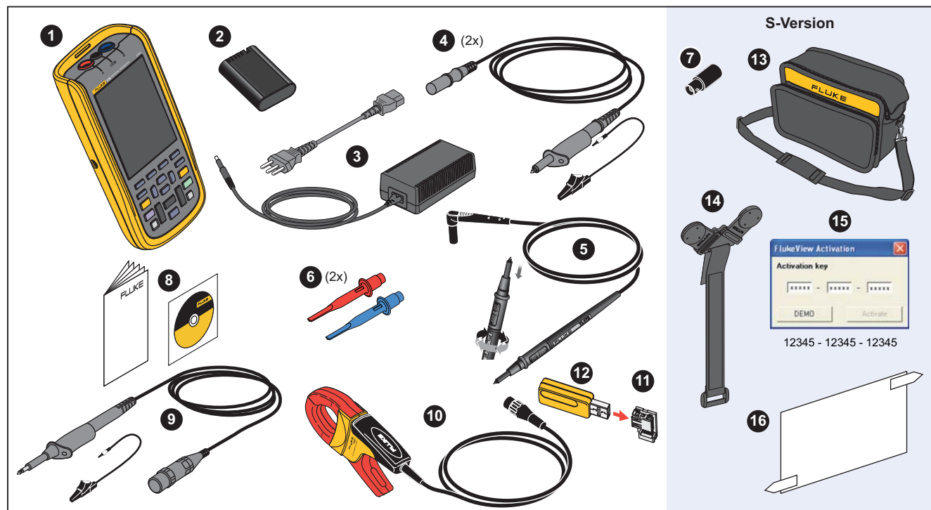
Figura 1. Kit del Instrumento de comprobación
