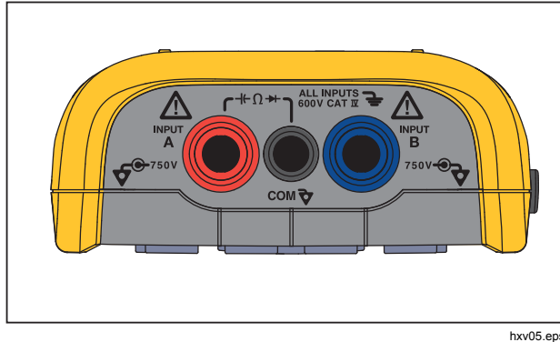
Figura 4. Conexiones de entrada para la medición
