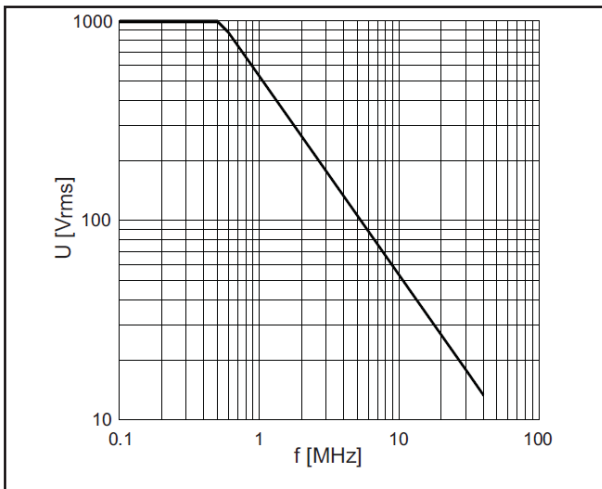
Figura 15. Tensión de entrada máx. frente a frecuencia para BB120 y STL120-IV
