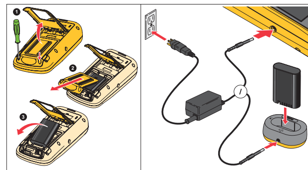
Figura 2. Carga de baterías
