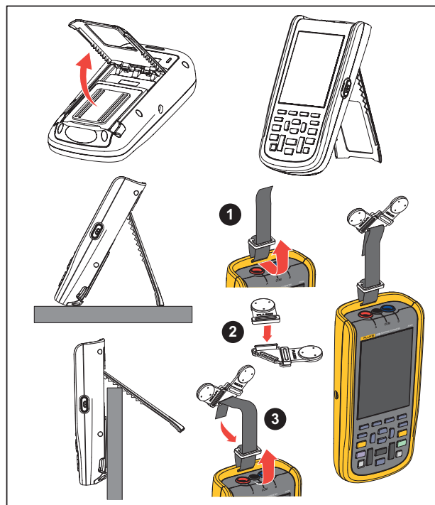
Figura 5. Soporte inclinable y colgador
