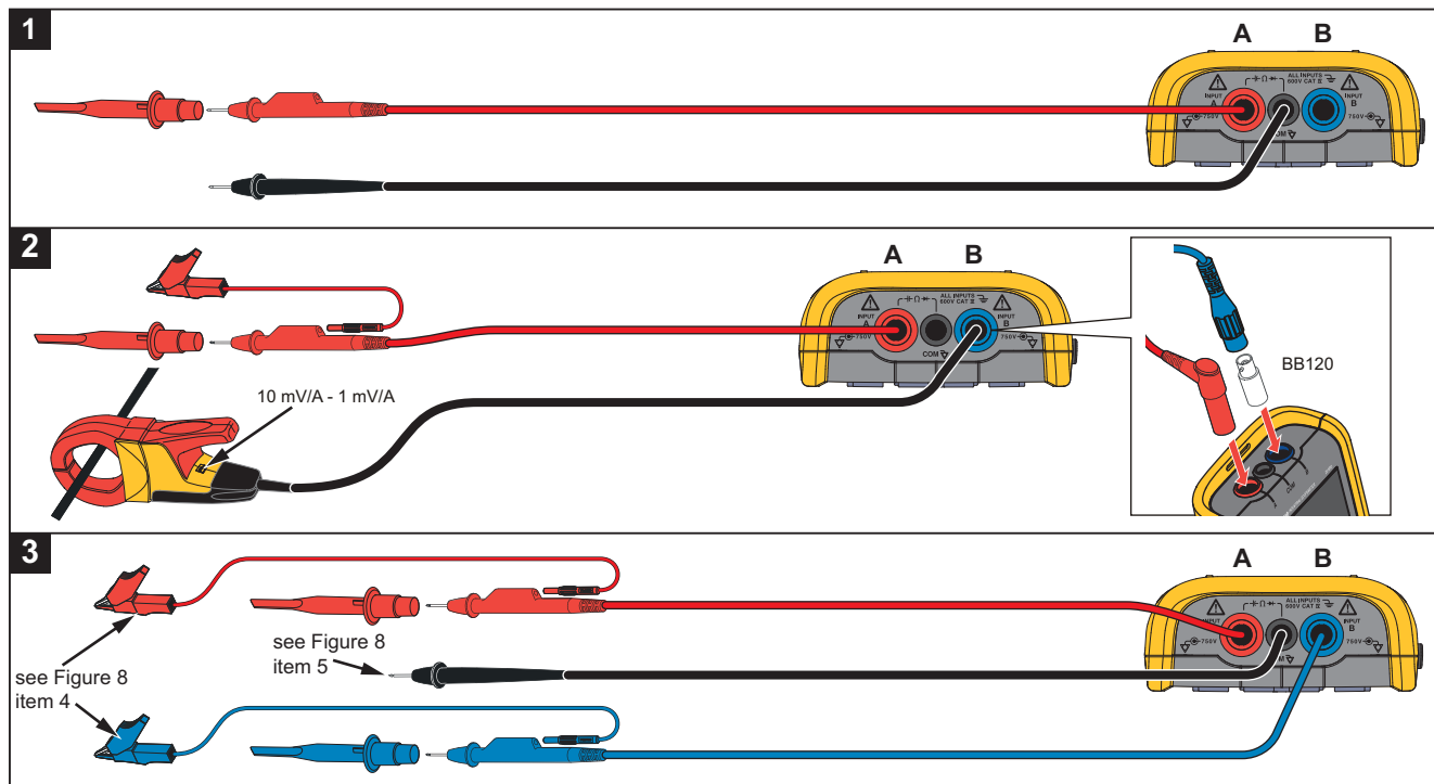
Figura 7. Configuración de medición
