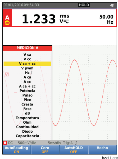
Figura 10. Función AutoReading (Lectura automática)
