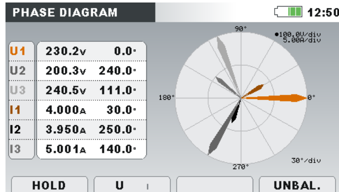
Figura 3.36: Pantalla de diagrama de fase
