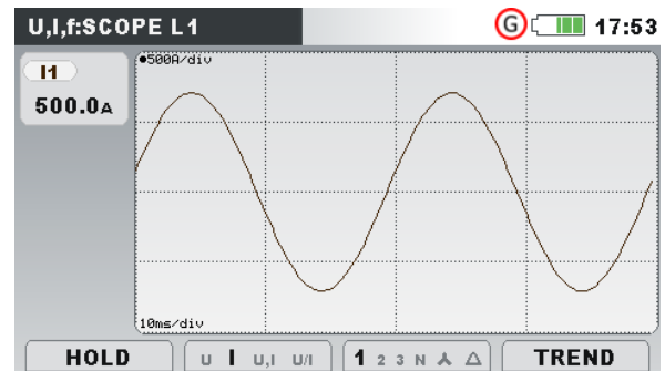
Figura 3.13: Forma de onda de solo corriente
