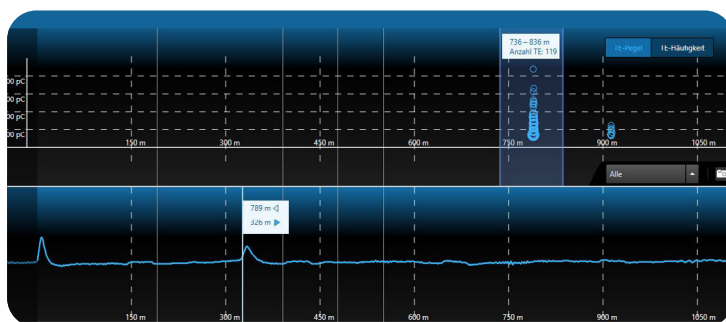
Visualización combinada de localización y evaluación DP ↑
