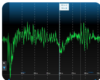
Señal DP con interferencias ↑
